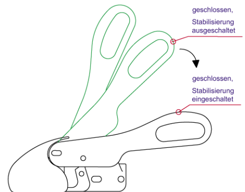
Bild 5: Stabilisierung einschalten
